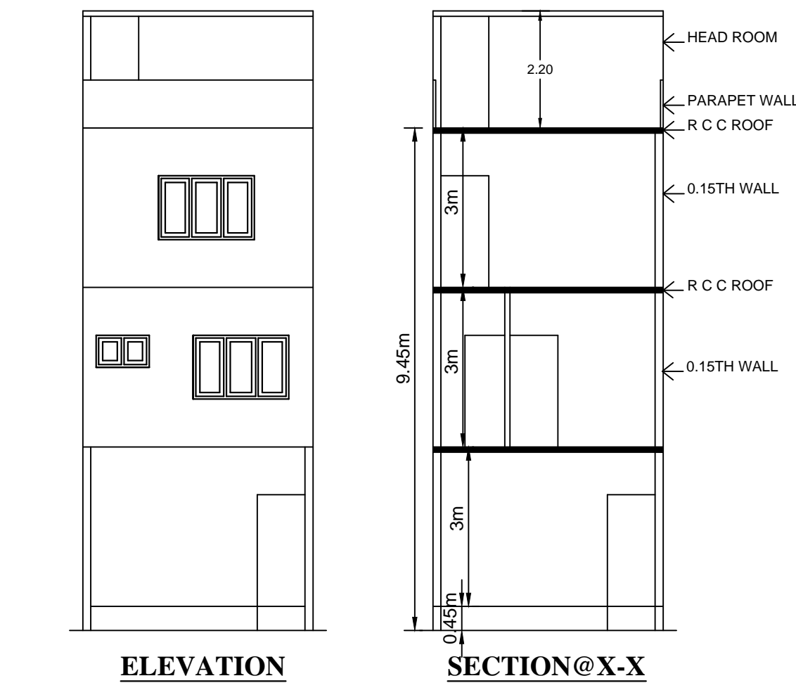
ELEVATION
